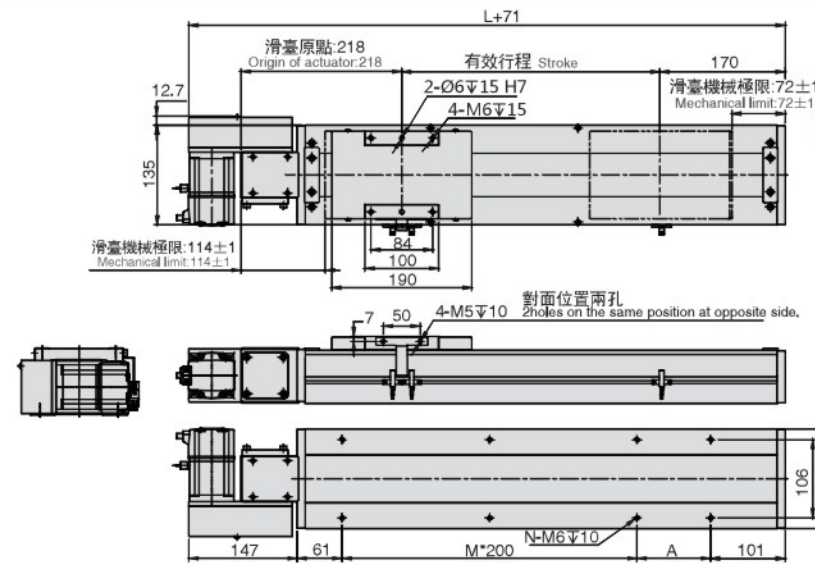
BL 马达左折 Motor Left Side
