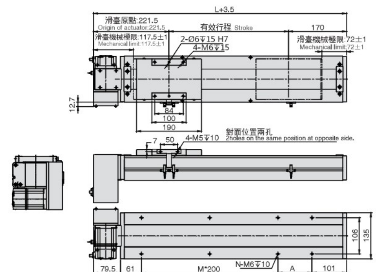
RD 马达右下折 Motor Right Lower Side
