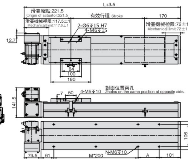
LU 马达左上折 Motor Left Upper Side
