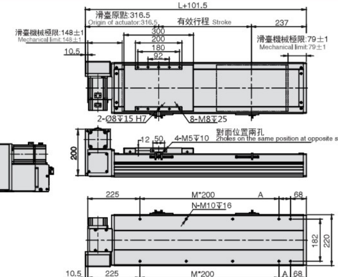
LU 马达左上折 Motor Left Upper Side
