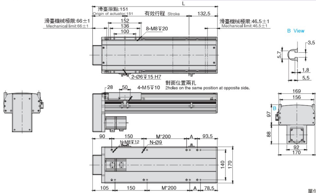
BM 马达下折 Motor Bottom Side
