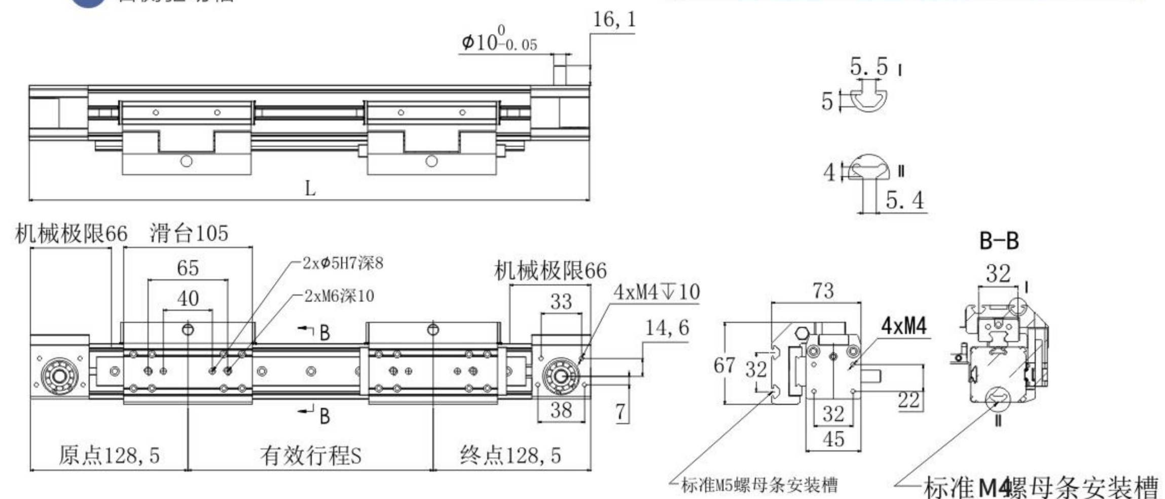
● 右侧驱动轴
