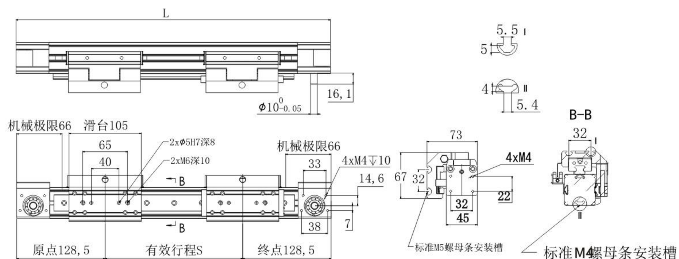
● 左侧驱动轴
