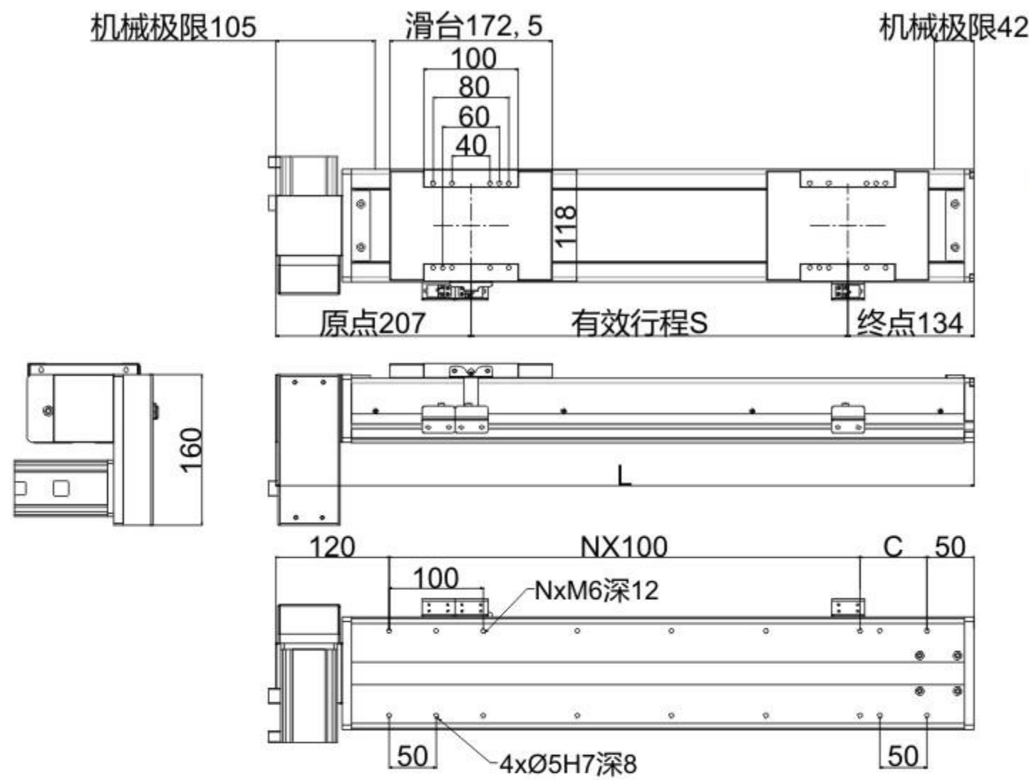
RD 马达右下折 Motor Right Lower Side
