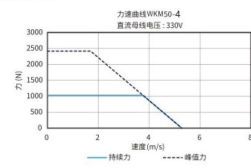
力-速度曲线
