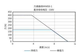
力-速度曲线
