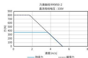
力-速度曲线
