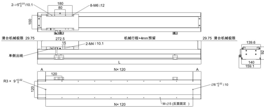
• MNK140-MK12 尺寸参数
