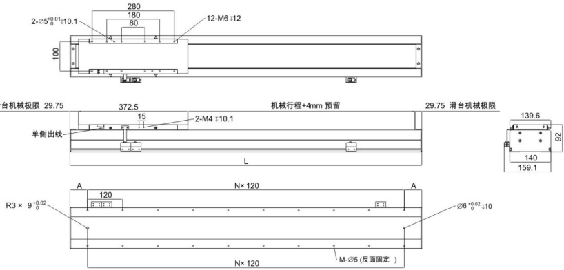
• MNK140-MK13 尺寸参数
